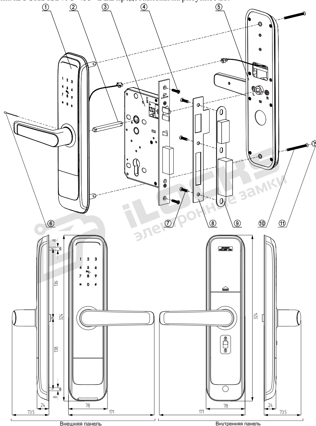
Рисунок №1 – Структурная схема (спецификация) и габаритные характеристики замков типа IS240C 433+BLE
